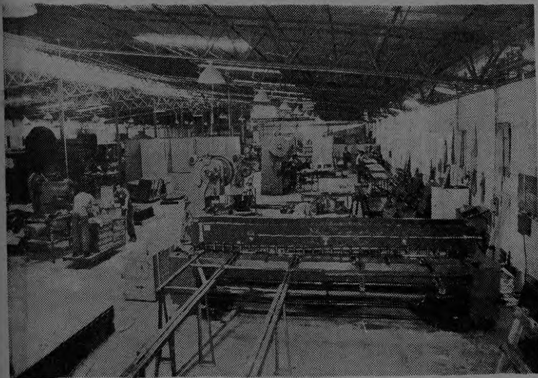
Vista parcial de la Planta en donde se fabrican los GABINETES, PUERTAS y demás partes metálicas de los refrigeradores.
