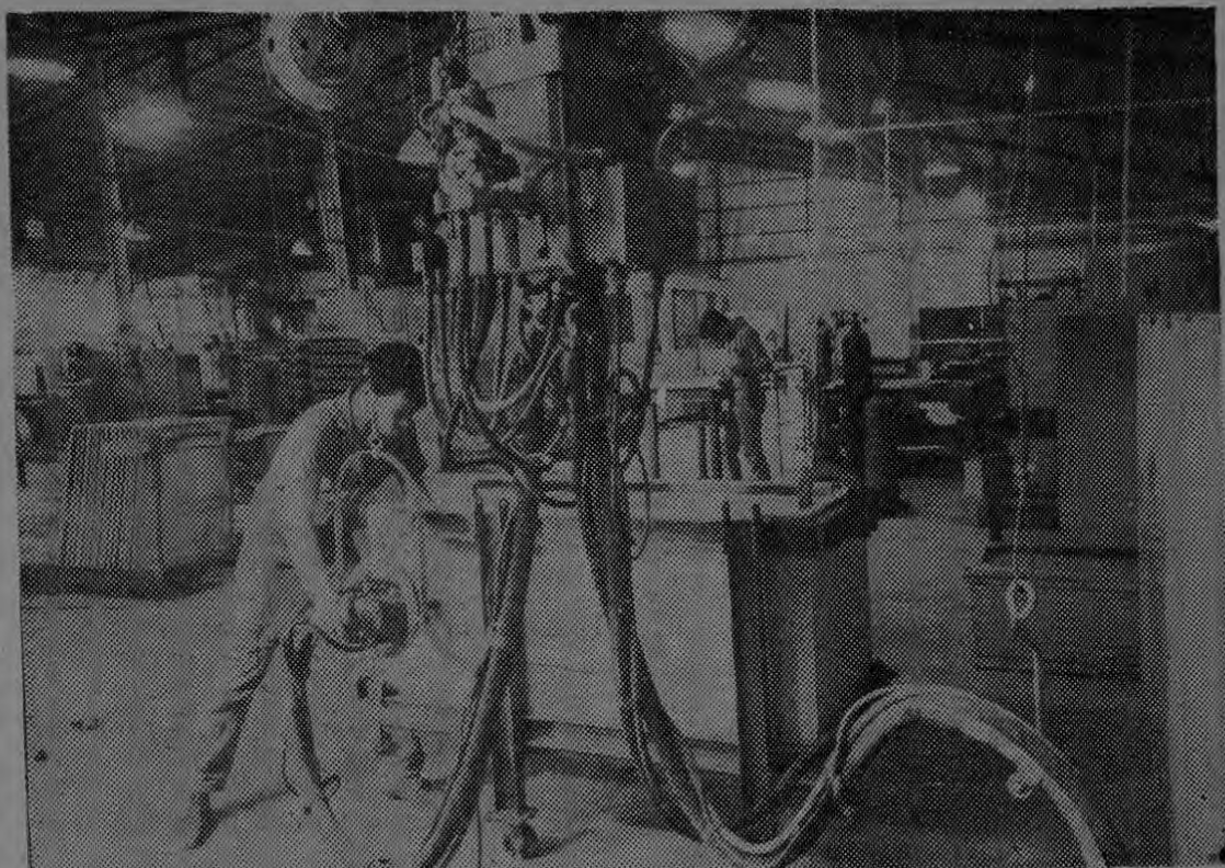
Equipo moderno en su maravilloso funcionamiento de "Soldadura de Puntos", con lo que se da forma al mueble del REFRIGERADOR DE TIPO DOMESTICO
